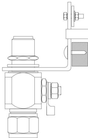
Рисунок 3.2 Крепление грозозащитника
