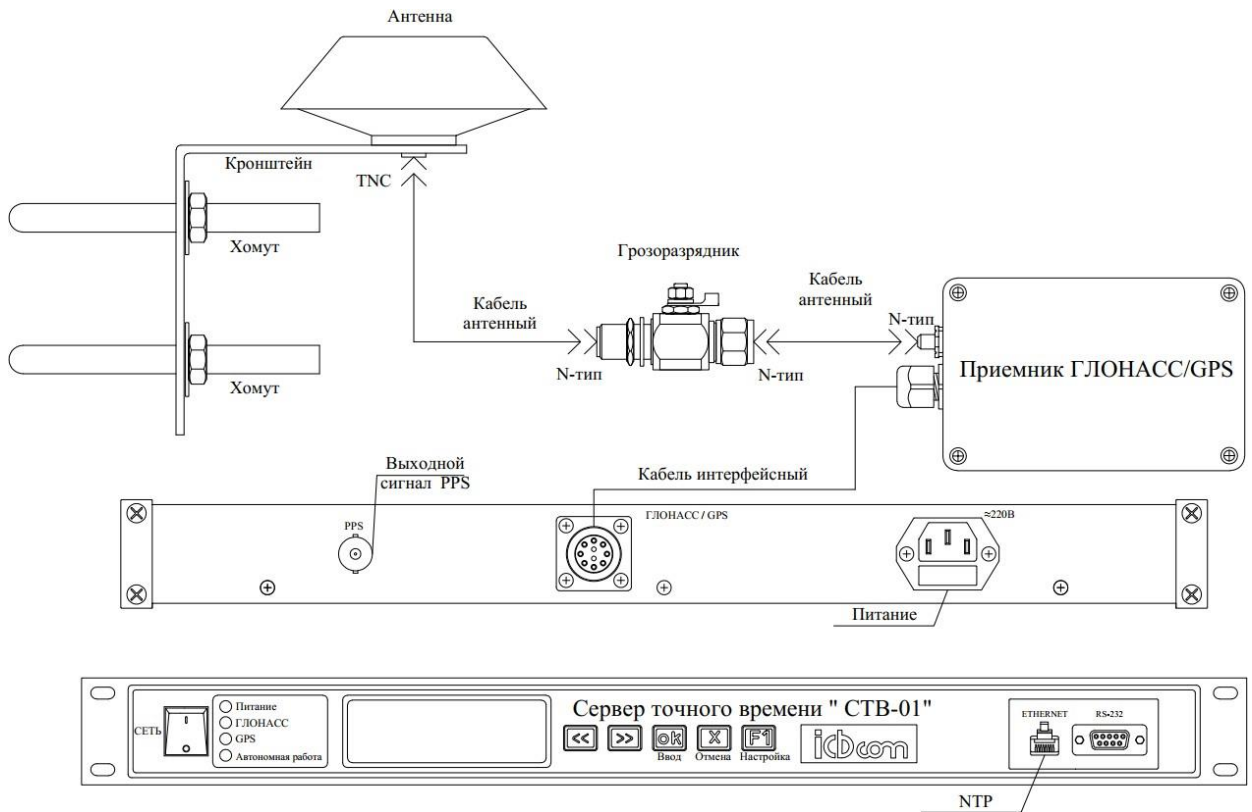
Рисунок 3.1 Схема соединения узлов СТВ-01 (19")
