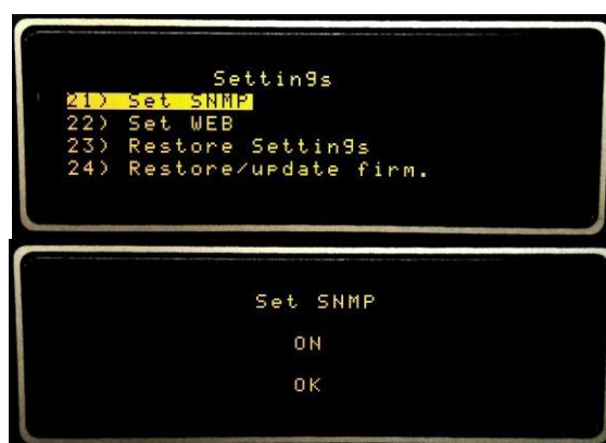
Рисунок 21 — Настройка SNMP
