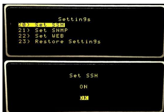
Рисунок 20 — Настройка SSH
