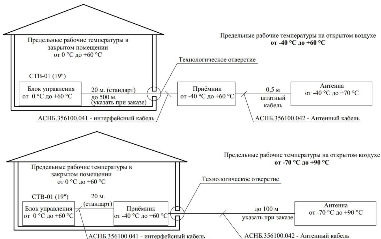
Рисунок 1.1 Подключение СТВ-01(19”) в различных температурных диапазонах.
