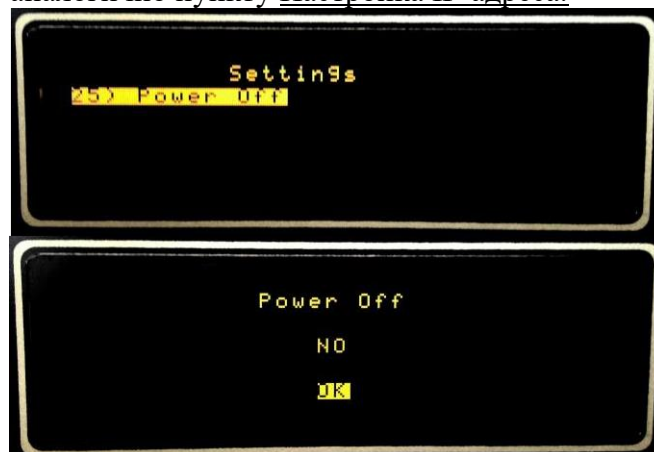
Рисунок 25 — Отключение системы
